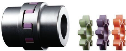
ROTEX® POLY
